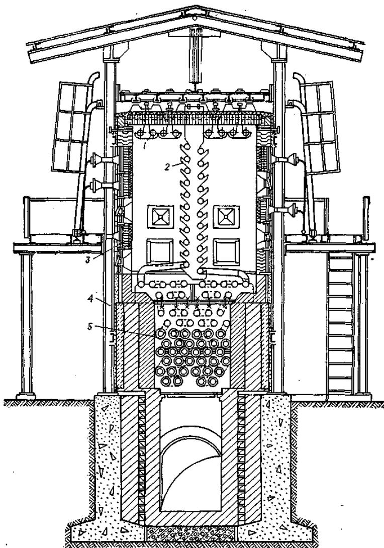
Рис.5. Трубчатая печь пиролиза с экранами двустороннего облучения: 1 — потолочный экран; 2 — экран двустороннего облучения; 3 — панельные горелки; 4 — каркас; 5 — конвекционная камера.
